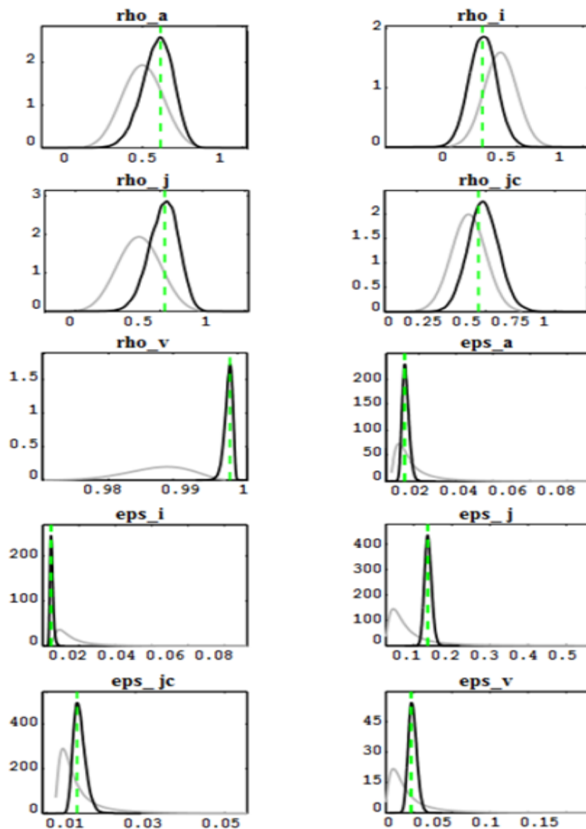
شکل ۲. چگالی پیشین و پسین پارامترهای برآورد شده مدل ماخذ: یافته‌های پژوهش
