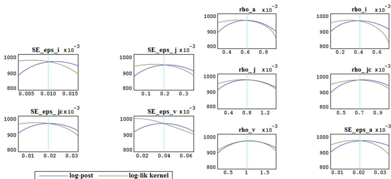
شکل ۱. بررسی نمای محاسبه شده پارامترهای برآوردشده مدل
